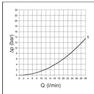
Áramlási ellenállás
